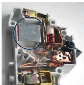
Une copie de disjoncteur Hager avec une chambre de coupure en acier massif.
