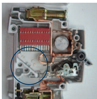
Une contrefaçon de disjoncteur Hager sans déclencheur magnétique ni bilame.
